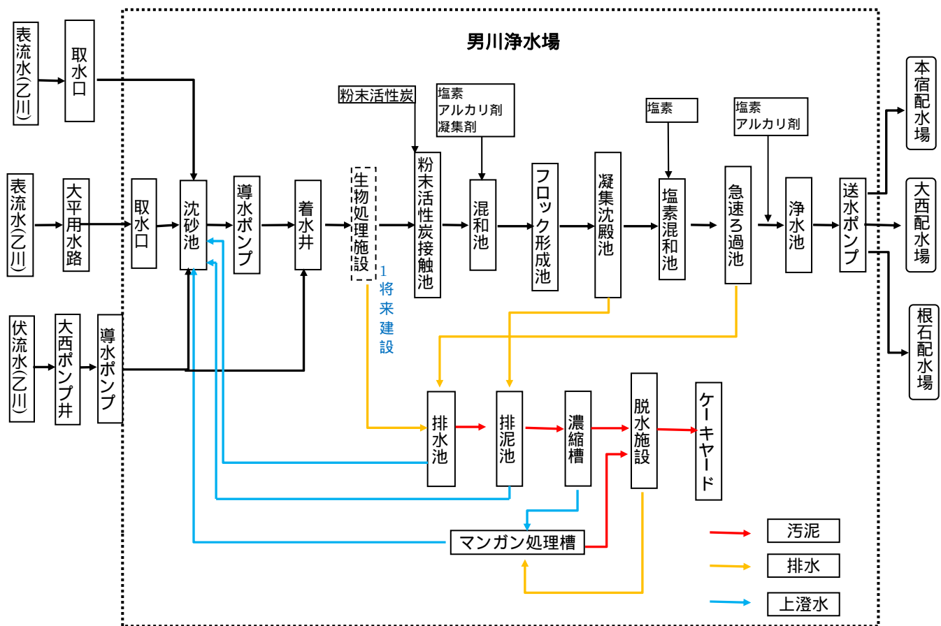
図 2 - 1 男川浄水場廻り処理フロー
