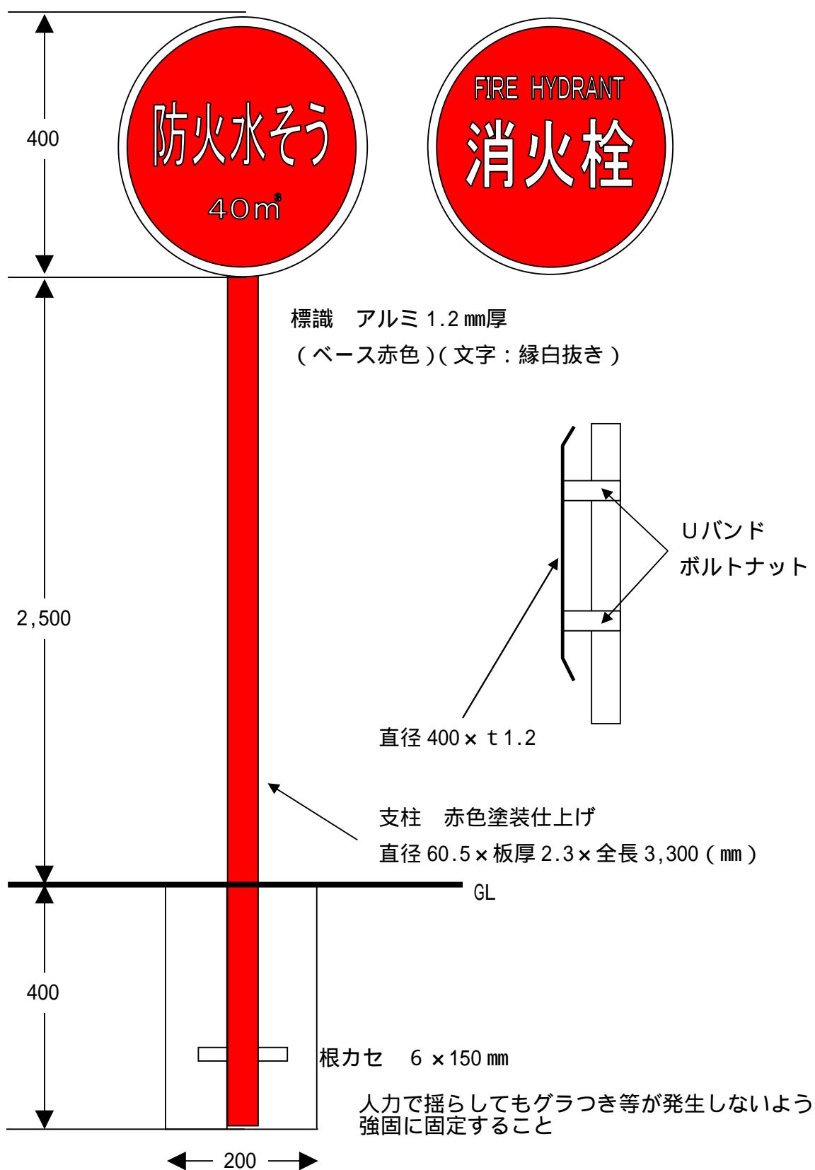
防火水槽・消火栓標識規格図
