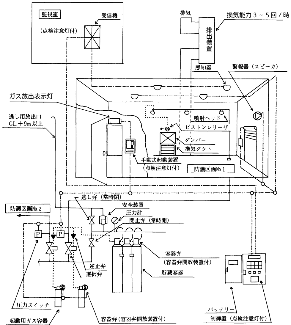
(1) 不活性ガス消火設備系統図 (例1)
