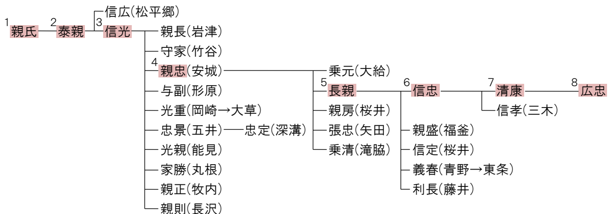
図3-7 松平八代系図
