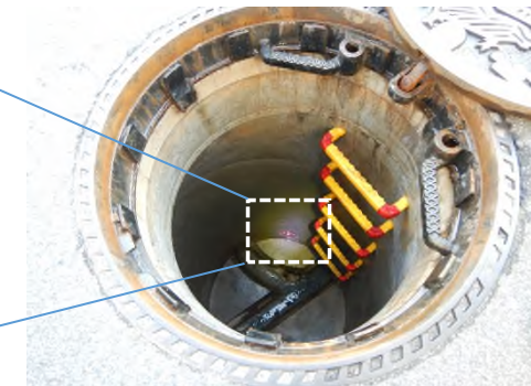
マンホール浮上防止の状況
