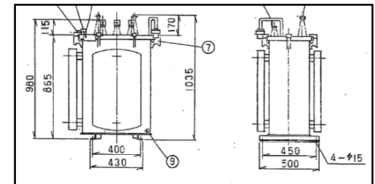
トランス図
