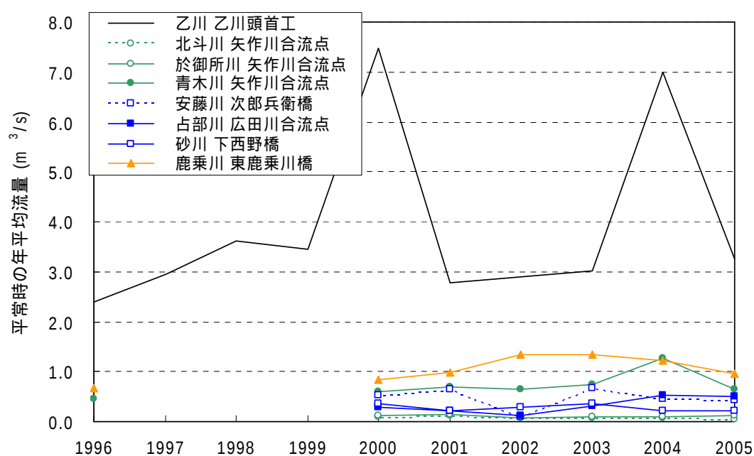
図 2-8 岡崎市の主な河川の流量の観測結果
