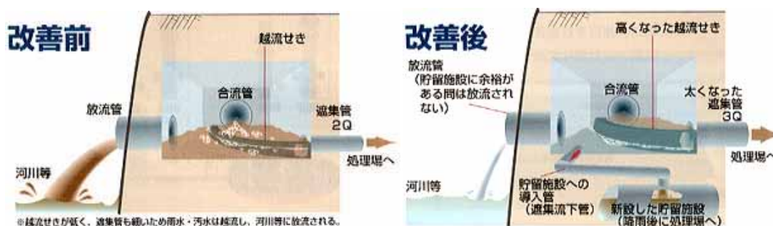
図 5-9 合流式下水道改善のイメージ (出典: 東京都 HP)
