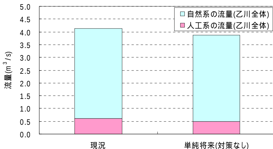
図 6-6 乙川下流ブロックの現況と単純将来の河川の流量(占部用水取水点)
