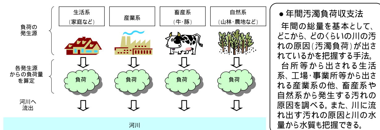
図 6-2 年間汚濁負荷収支のイメージ図
