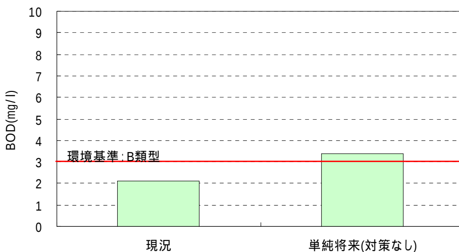
図 6-7 乙川下流ブロックの現況と単純将来の河川の水質(BOD75%値)
