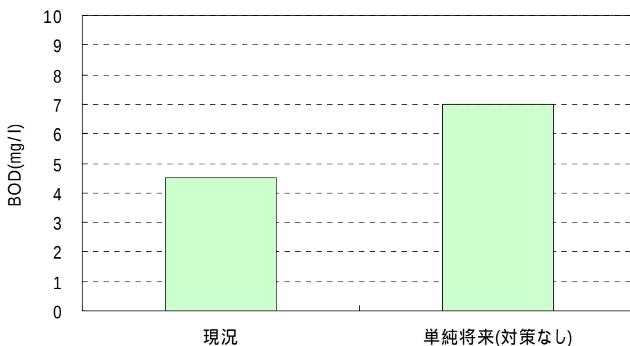
図 6-13 広田川・安藤川ブロックの現況と単純将来の河川の水質 (BOD75%値)
