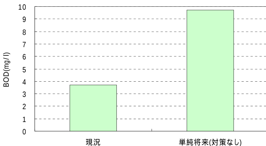
図 6-10 青木川・郡界川ブロックの現況と単純将来の河川の水質(BOD75%値)
