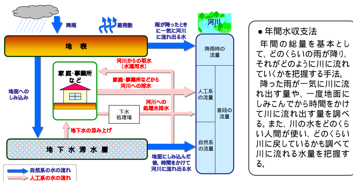
図 6-1 年間水収支のイメージ図
