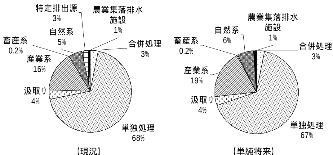
図 6-8 乙川下流ブロックの現況と単純将来の汚濁負荷の内訳
