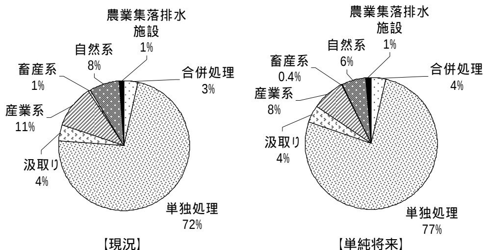
図 6-11 青木川・郡界川ブロックの現況と単純将来の汚濁負荷の内訳
