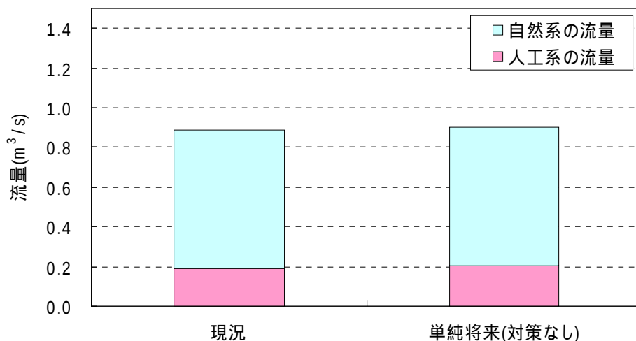
図 6-9 青木川・郡界川ブロックの現況と単純将来の河川の流量(青木川 + 北斗川 + 於御所川)
