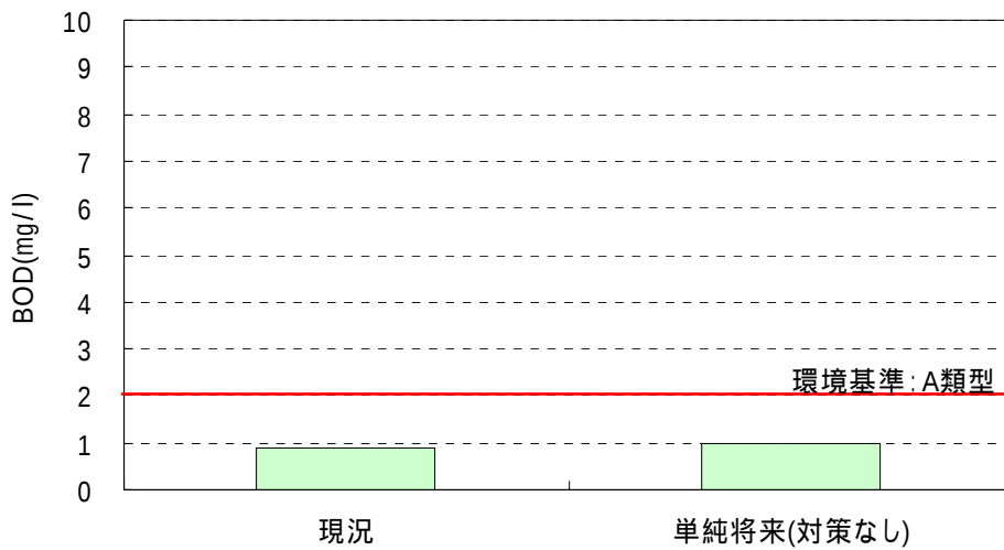
図 6-4 乙川上流ブロックの現況と単純将来の河川の水質(BOD75%値)
