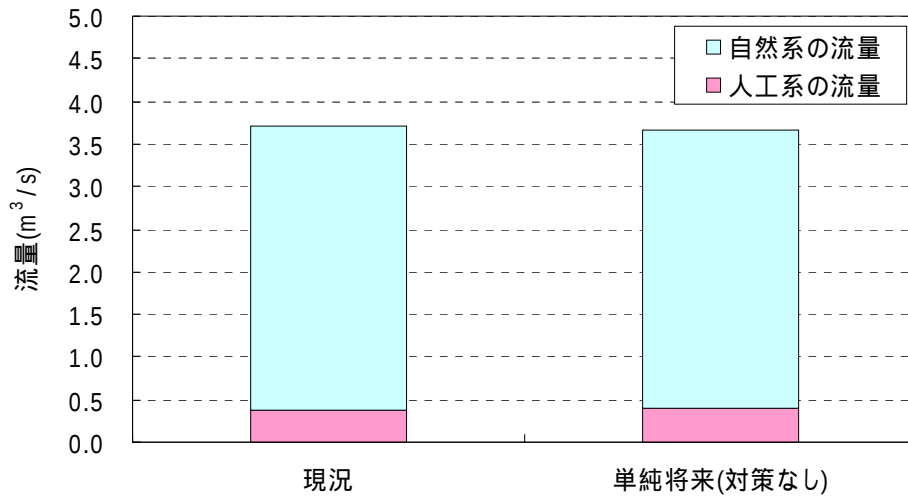
図 6-3 乙川上流ブロックの現況と単純将来の河川の流量(乙川 + 男川)
