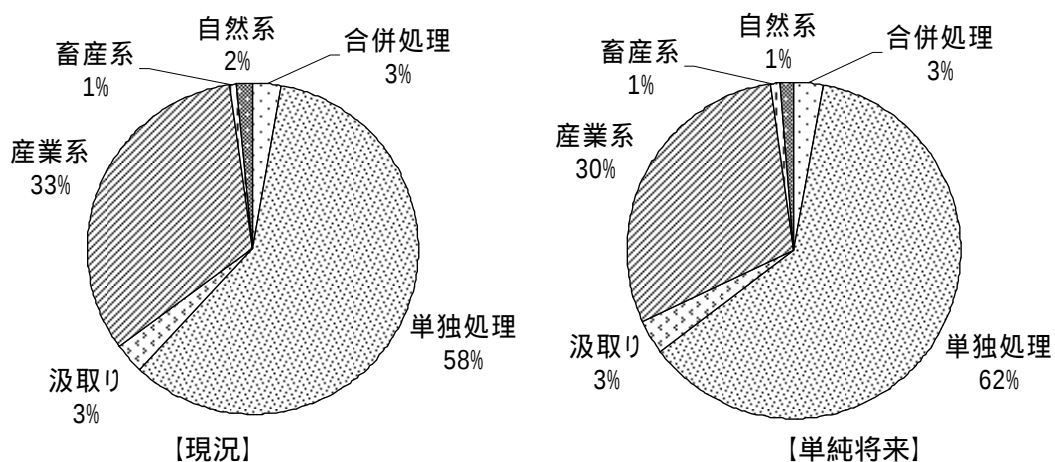
図 6-17 鹿乗川ブロックの現況と単純将来の汚濁負荷の内訳
