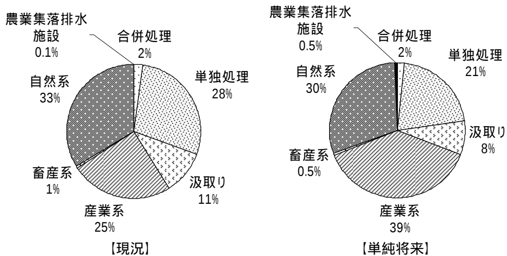
図 6-5 乙川上流ブロックの現況と単純将来の汚濁負荷の内訳
