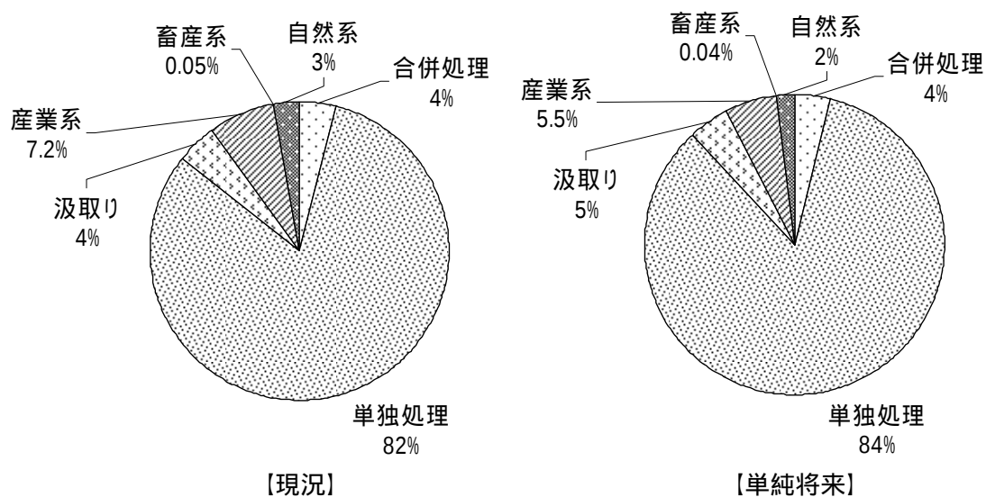
図 6-14 広田川・安藤川ブロックの現況と単純将来の汚濁負荷の内訳
