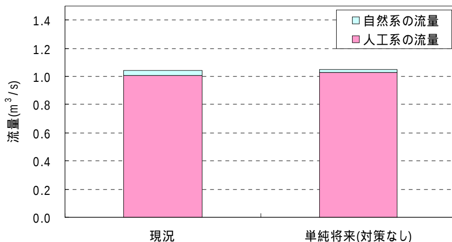
図 6-15 鹿乗川ブロックの現況と単純将来の河川の流量(東鹿乗橋)
