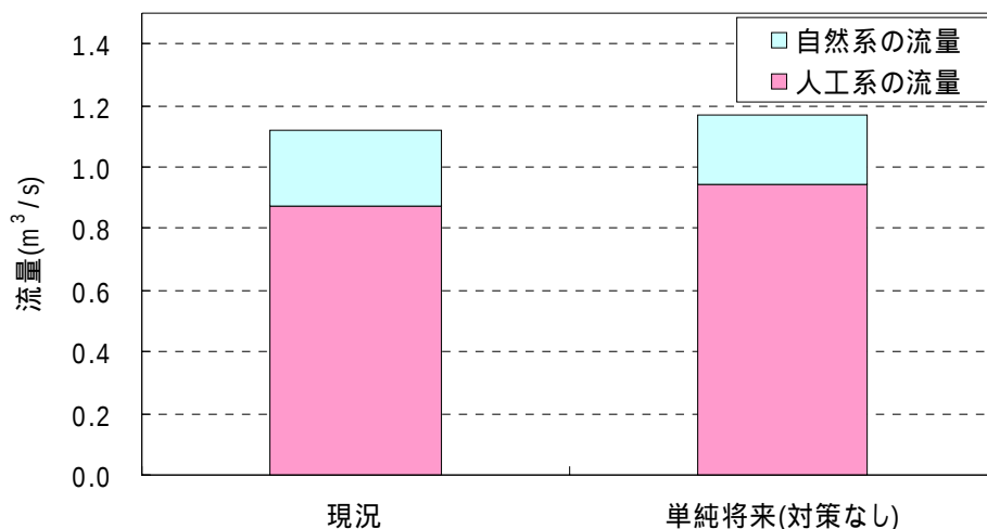
図 6-12 広田川・安藤川ブロックの現況と単純将来の河川の流量(安藤川 + 占部川 + 砂川)
