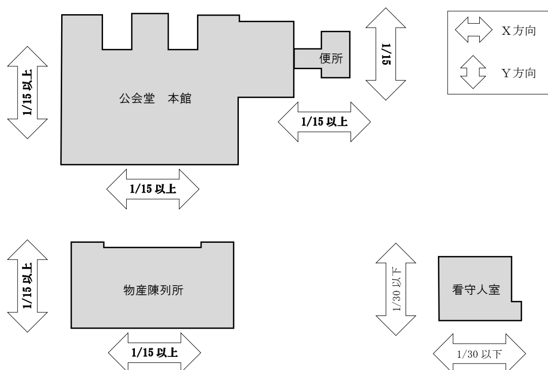
図 4-4 大地震時の建物の変形量
