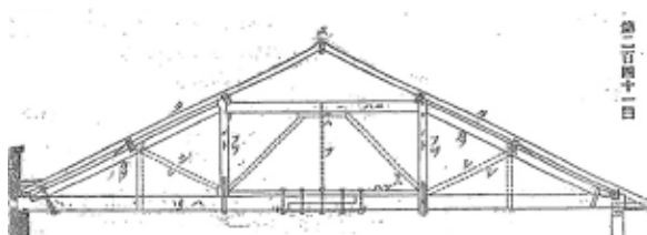
図 1-32 滝大吉『建築学講義録』収録の「二重梁小屋（Queen-Post Roof）」
