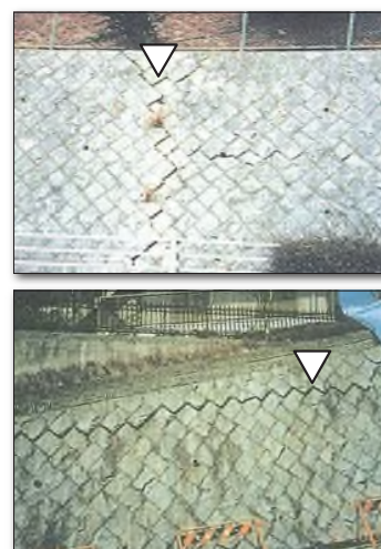
擁壁の割れ
