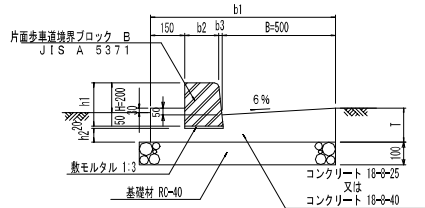
P L 1 型 側 溝 (セミフラット植樹帯部)
