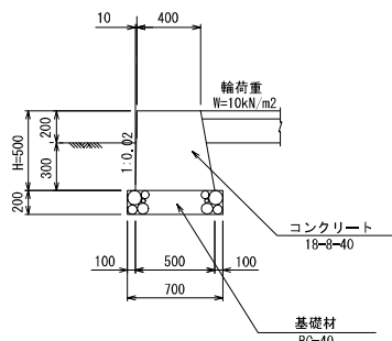
A - 1 型 H=500
