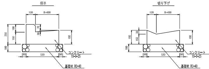
L 型 側 溝 (400型)
