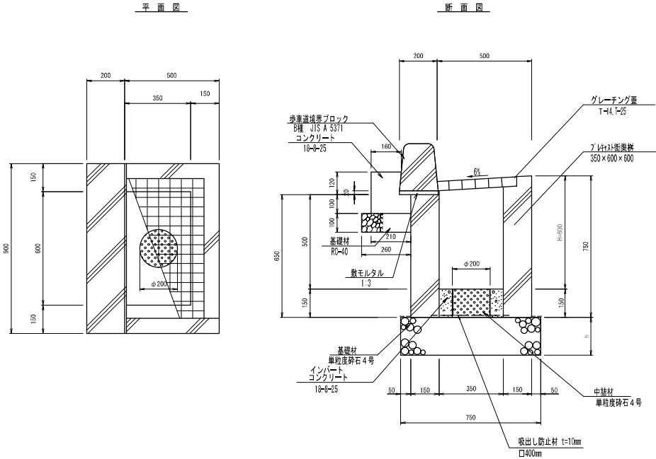
プレキャスト街渠枺 材料表
