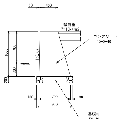
A - 2 型 H=1000
