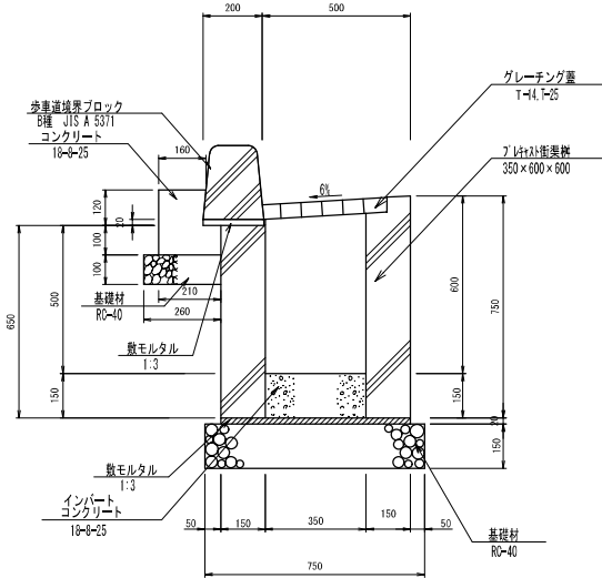
断面図
