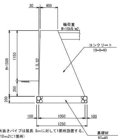
A - 3 型 H=1500
