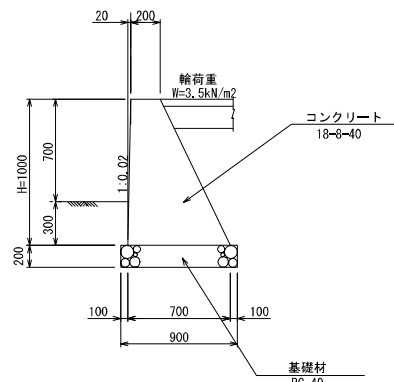
B - 2 型 H=1000
