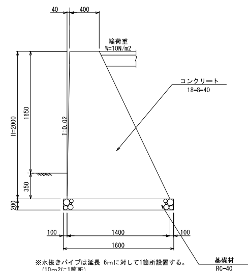
A - 4 型 H=2000
