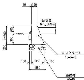
B - 1 型 H=500
