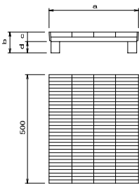
グレーチング蓋
