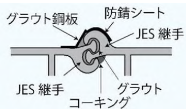
JES継手構造
