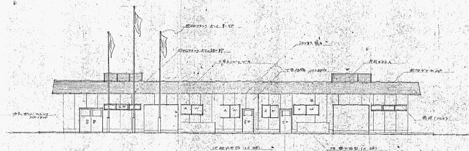
南面立面图 1/100
