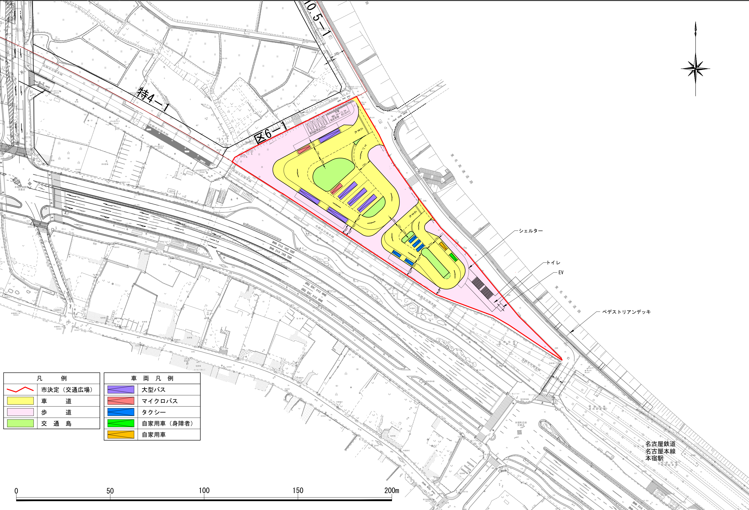
＜参考図＞西三河都市計画交通広場の変更（岡崎市決定）都市計画交通広場 第4号本宿駅交通広場 平面図 S=1:1,000
