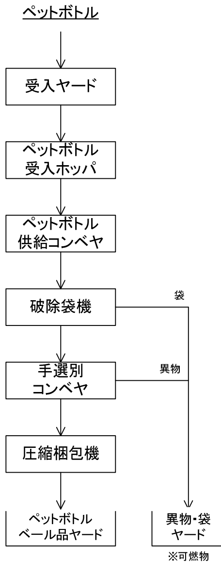
図 6 ペットボトルの基本処理フロー（ケース 2：前処理 + バール梱包）
