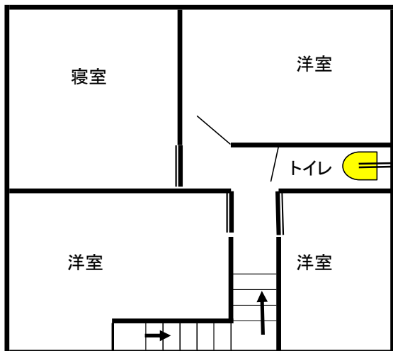
2F平面図
