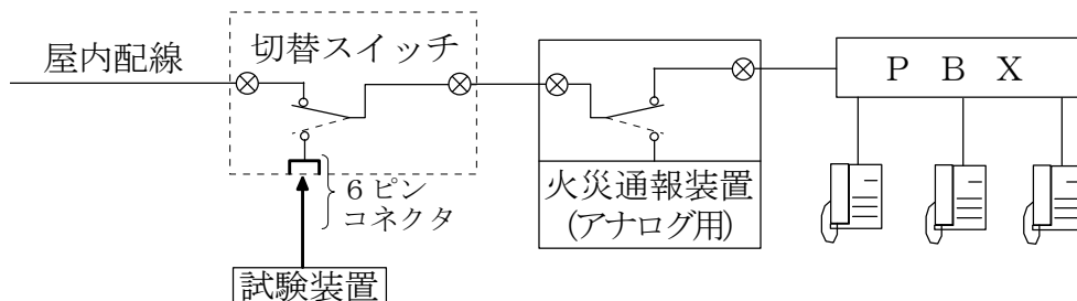
図 7 火災通報装置（アナログ用）と試験装置を接続する装置の設置方法
