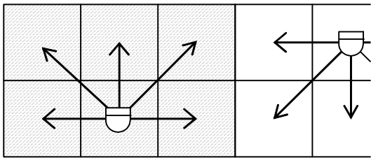
はり等の深さが0.4m以上1m未満 (煙感知器の場合は0.6m以上1m未満)
