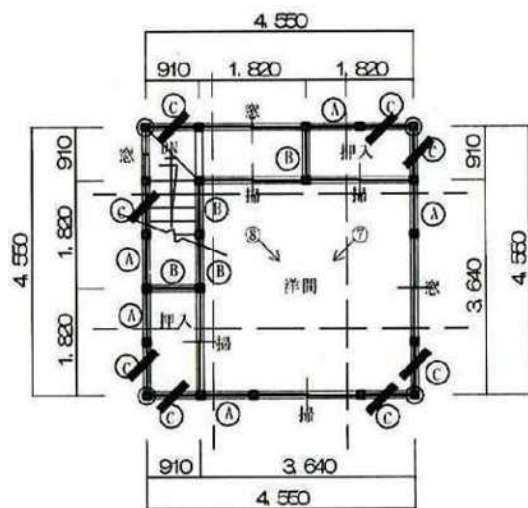
二階平面図 縮尺 1/100
