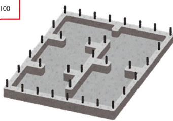
基礎の構造 コンクリート基礎と結合
