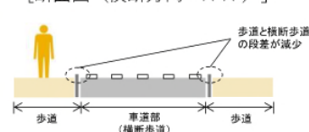
〔断面図 (横断方向：A-A')〕
