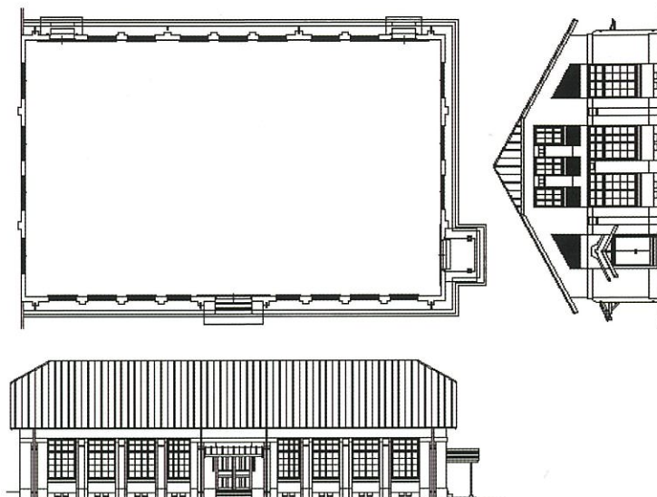
平面・立面図
