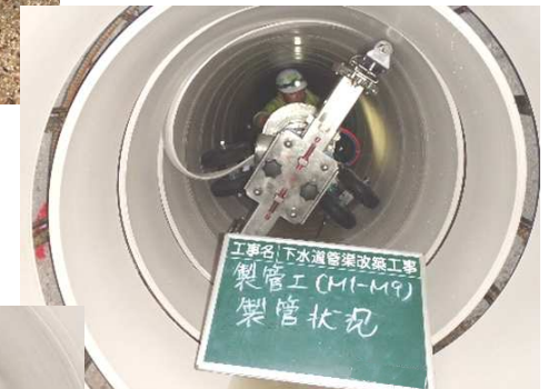
老朽化した下水道管の内側に新しい管を製作する状況
