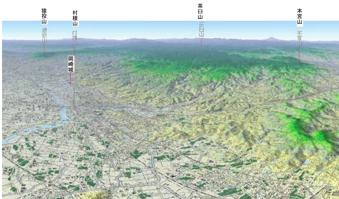
市域の地形の状況
