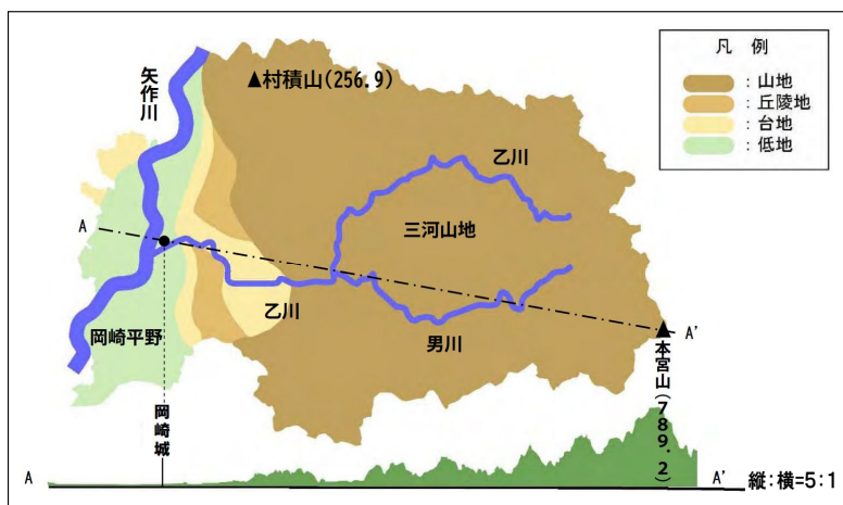
図1-1-3 岡崎市の高低差
