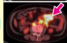
PET-CT 画像
