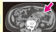
CT 画像
